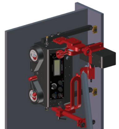
Kehlhaht-Schweißen mit Oszillator
